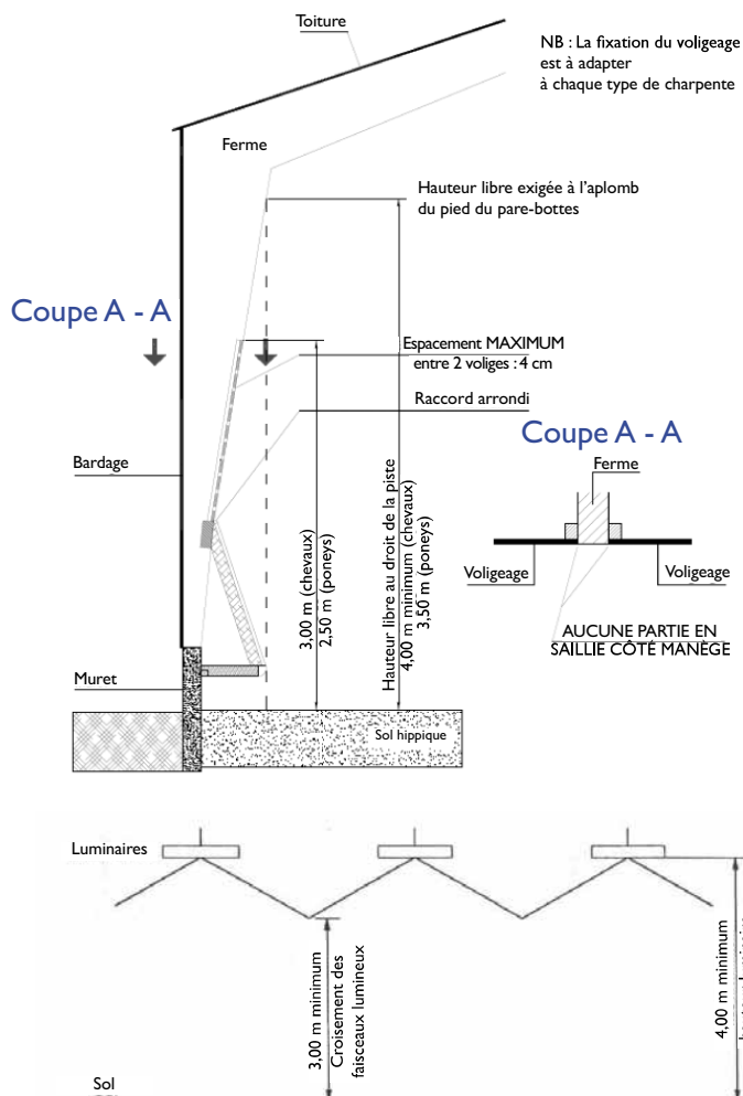
COUPE SUR PARE-BOTTES ET VOLIGEAGE
